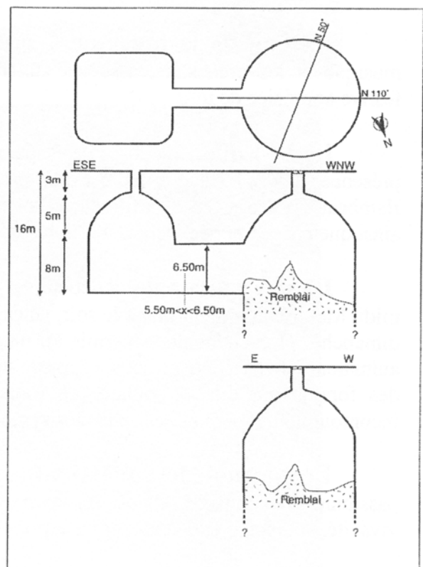
Figure 3 – Représentation en coupe des deux crayères. Le remblai, dans la seconde carrière, est réparti de manière hétérogène.
