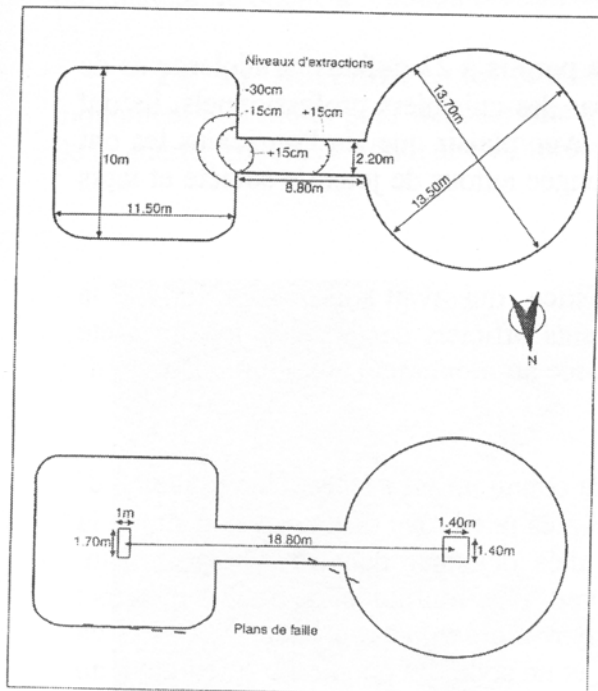
Figure 2 – Représentation en plan des deux carrières explorées. En haut, dimension des deux cavités. En bas, dimensions des puits d'accès et plans de faille.
